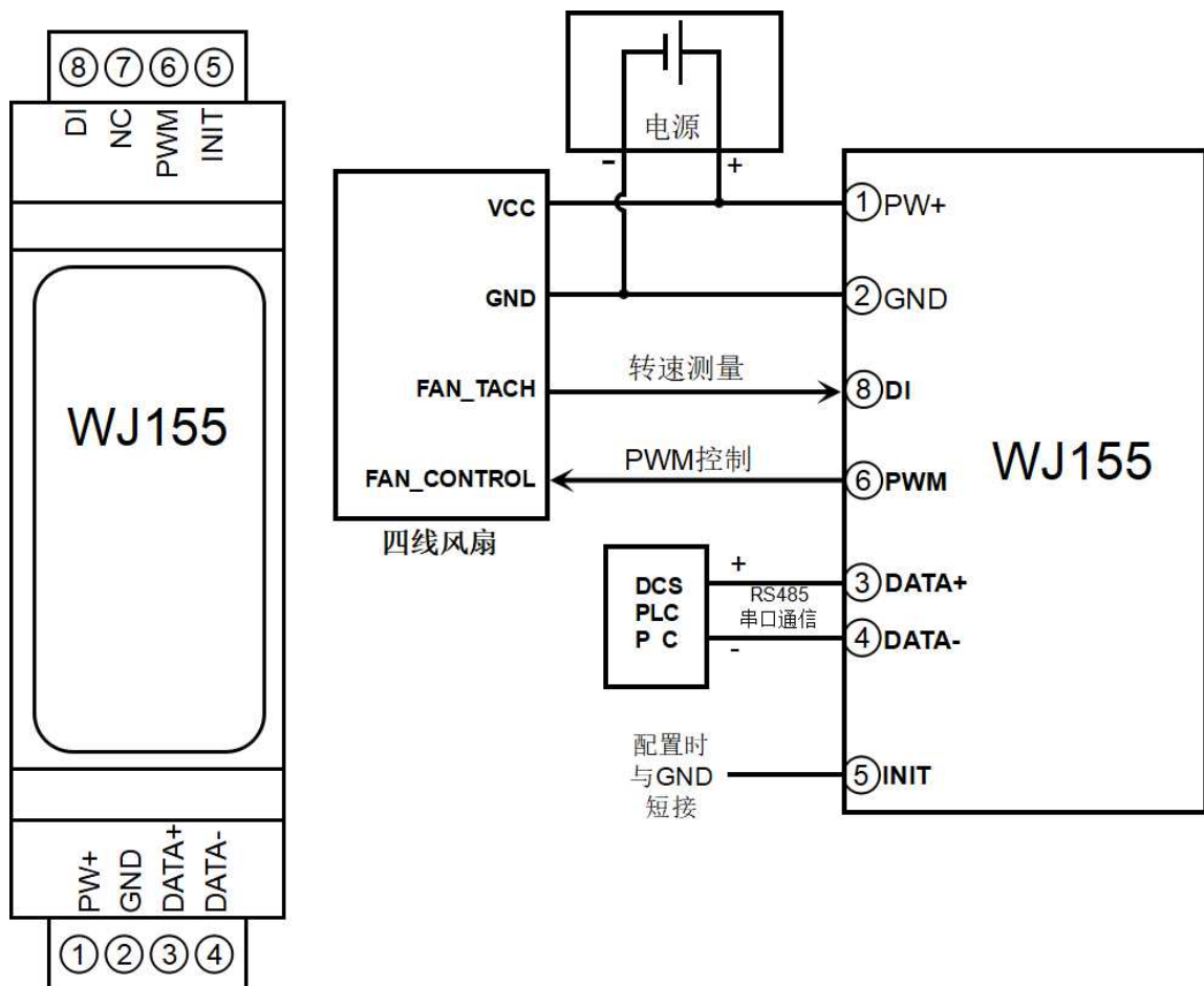
图3 WJ155 模块接线图
