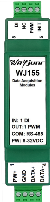
图1 WJ155 模块外观图
