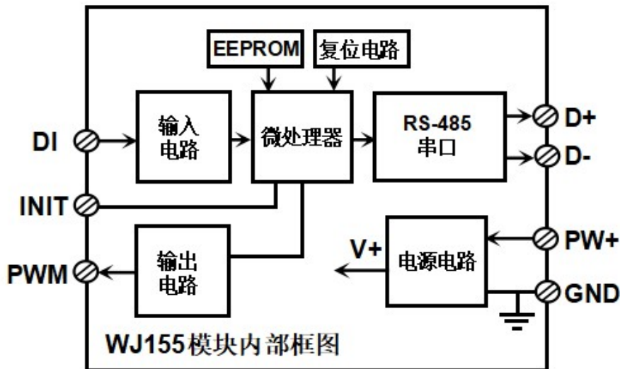
图2 WJ155 模块内部框图
